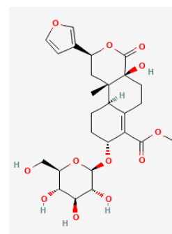
Cordifolisides D
