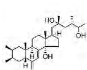
Ecdysterone
