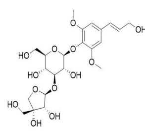
Cordifolisides A
