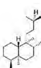
neo-clerodane(ent-clerodane)
