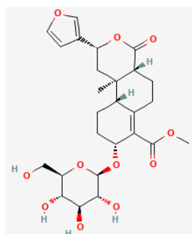
Cordifolisides B
