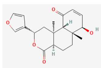
Tinosporone
