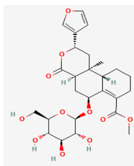
Cordifolisides C
