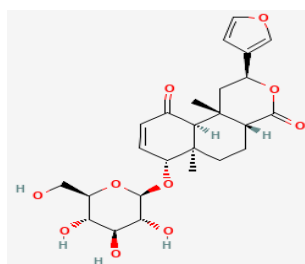
Tinosporaside
